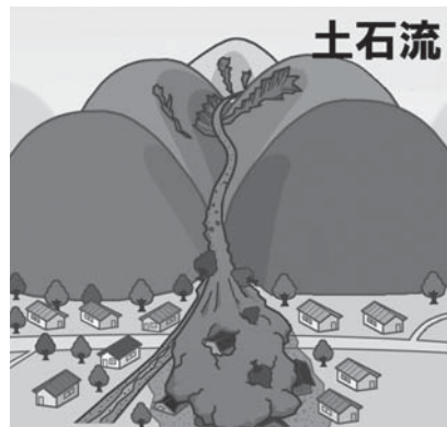
地すべり
