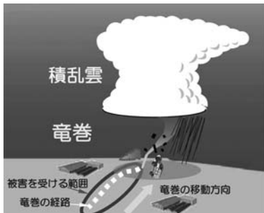
竜巻のイメージ図
