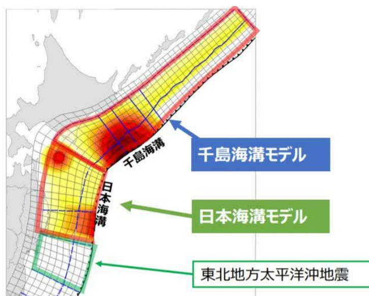
図3.1-2 想定する地震動
