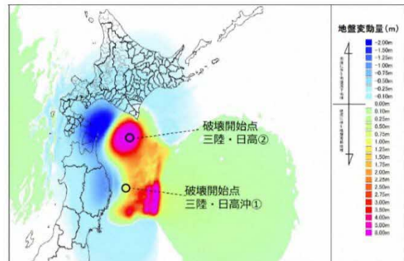
地盤変動量分布
