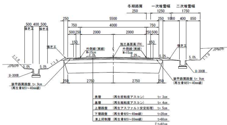
一般切土路肩(A)
