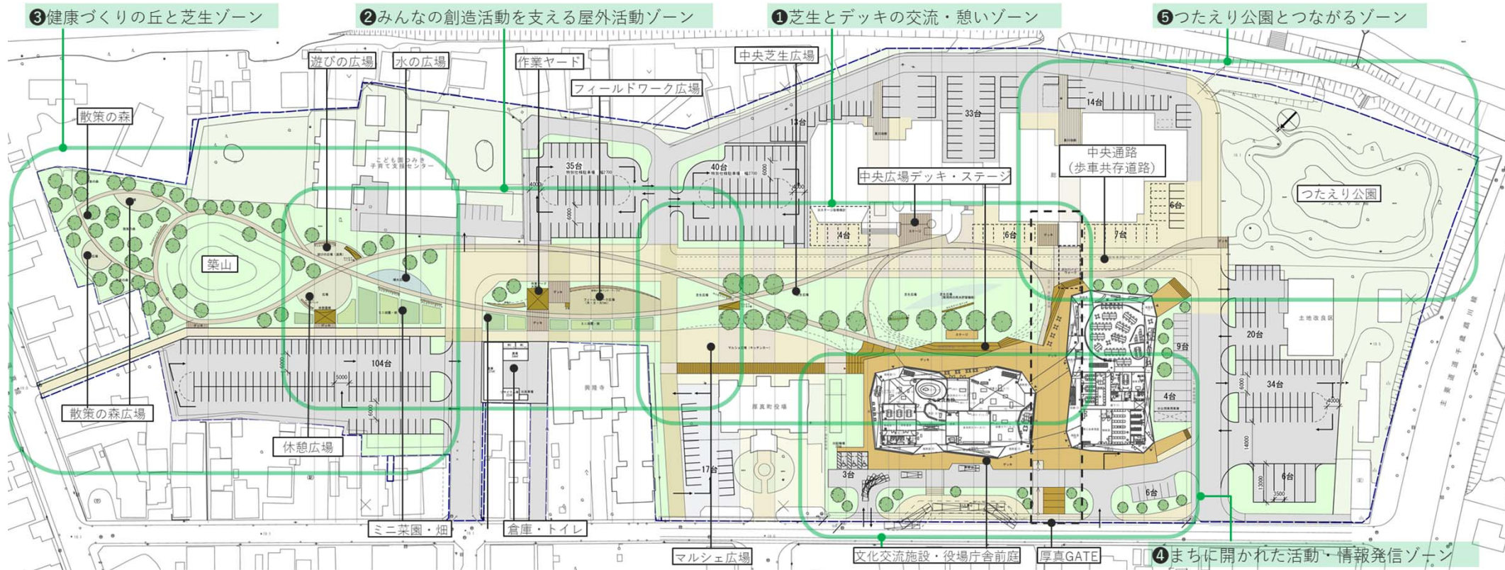
①立ち上がりデッキイメージ
