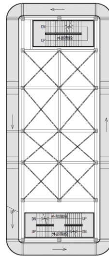
ピロティ階平面図
