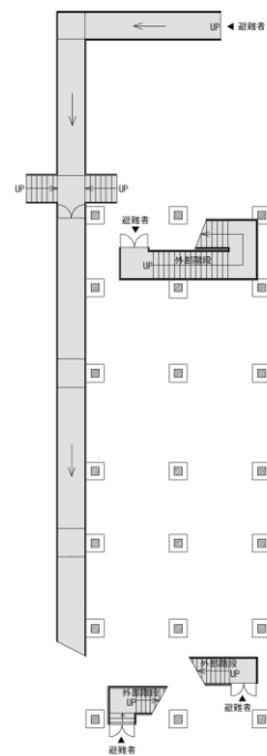
地上階平面図
