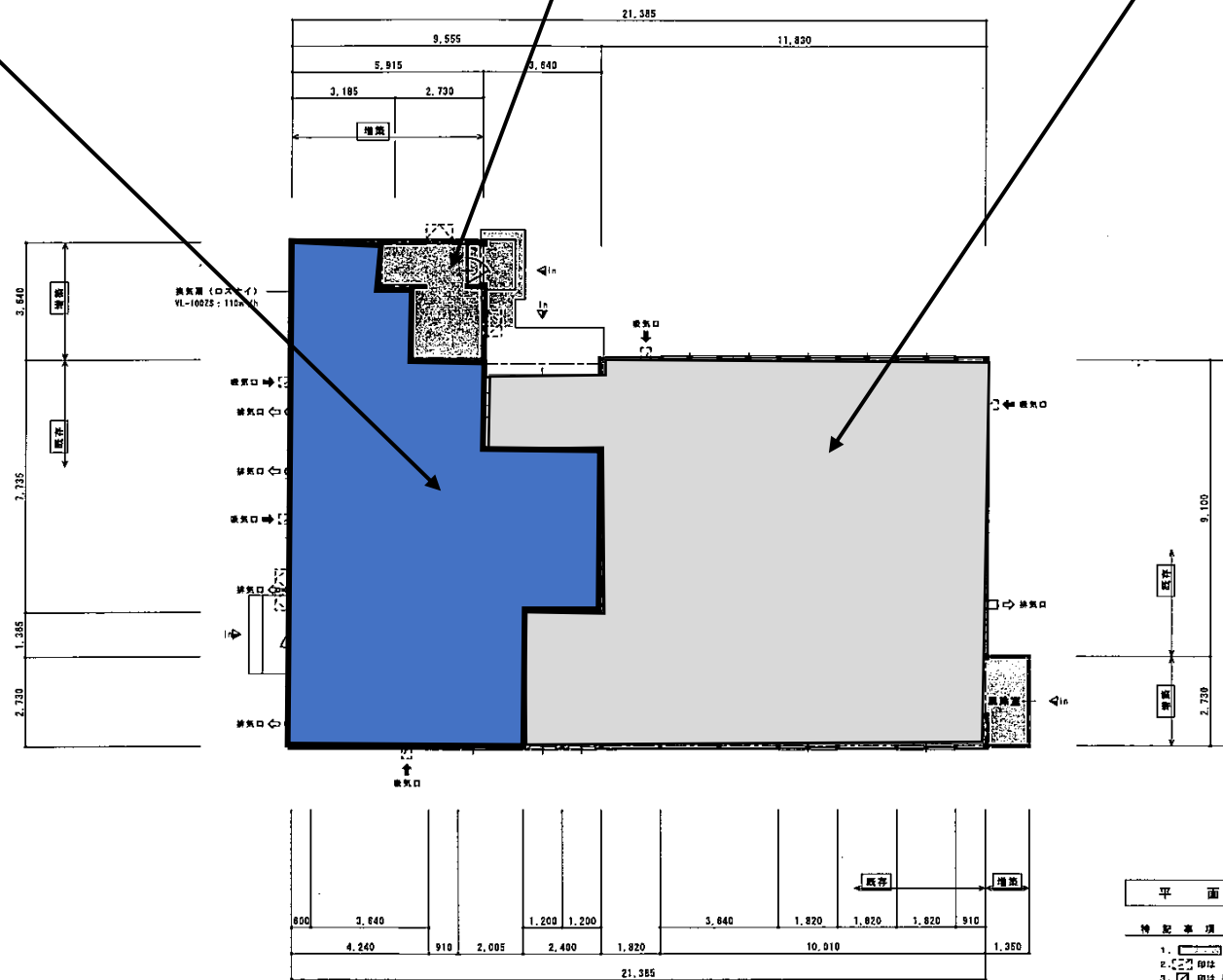
上厚真市街地店舗（旧資材店舗跡）平面図
