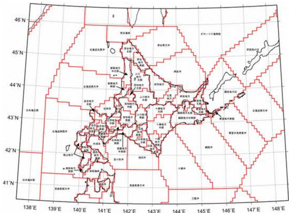
(イ) 震央地名
