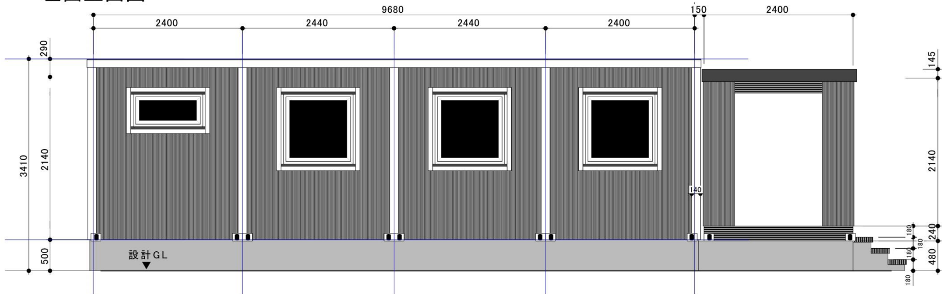
左面立面图
